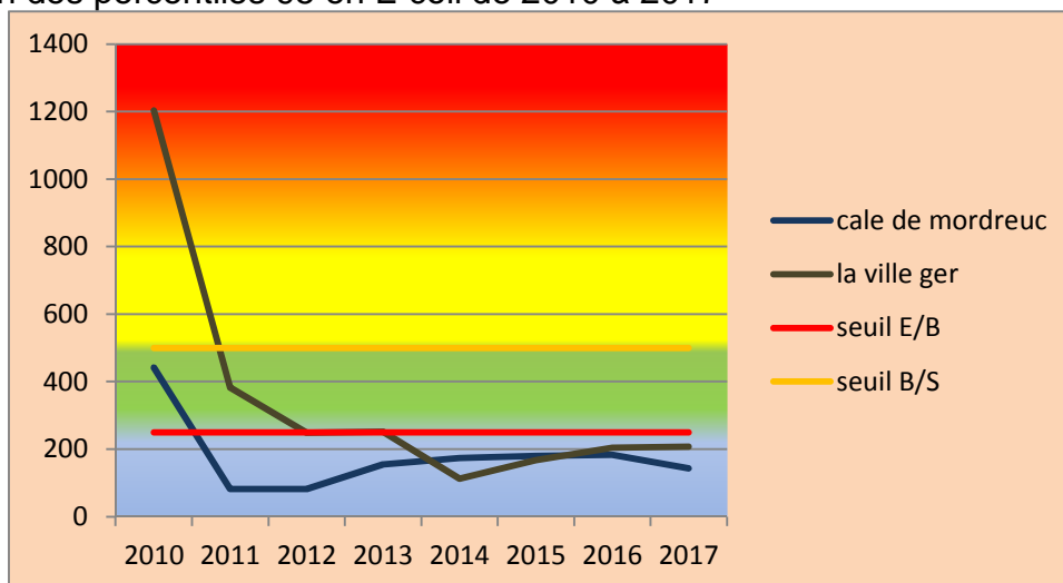
Evolution des percentiles 95 en E coli de 2010 à 2017
