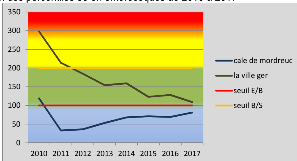
Evolution des percentiles 95 en entérocoques de 2010 à 2017
